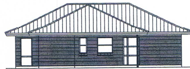
Facade mod nordøst
