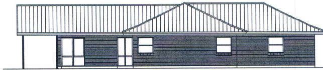
Facade mod sydøst
